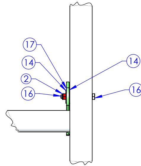
DÉTAIL A ECHELLE 1 : 5
